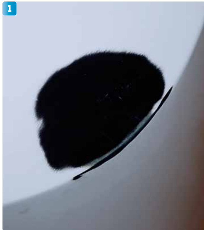
Laga skador i gelcoaten ovan vattenlinjen med ett fint polyesterspackel. Gammal gelcoat kan behöva grundmålas med epoxi.
